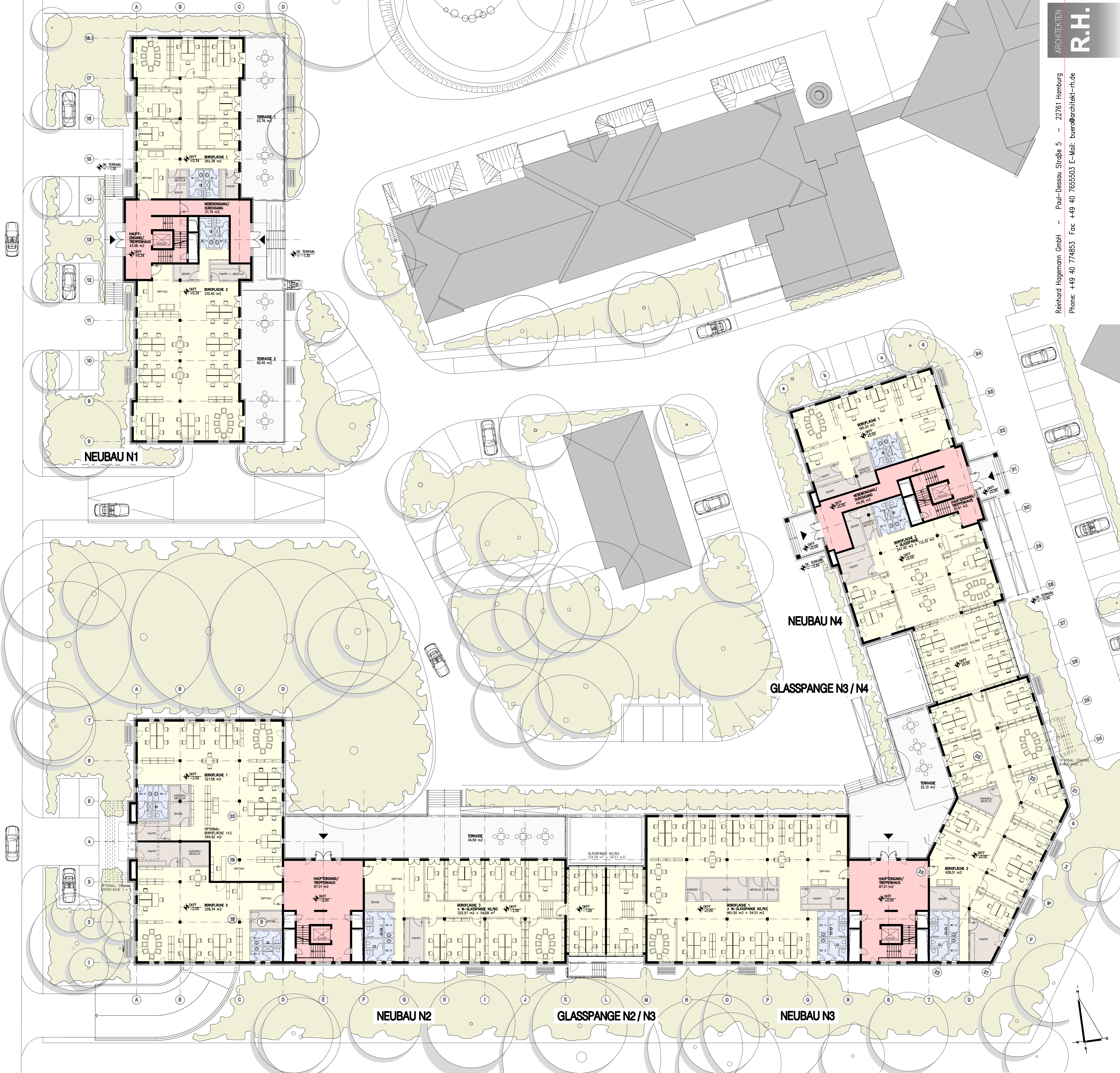
NEUBAU N1 - N4: GRUNDRISS ERDGESCHOSS
