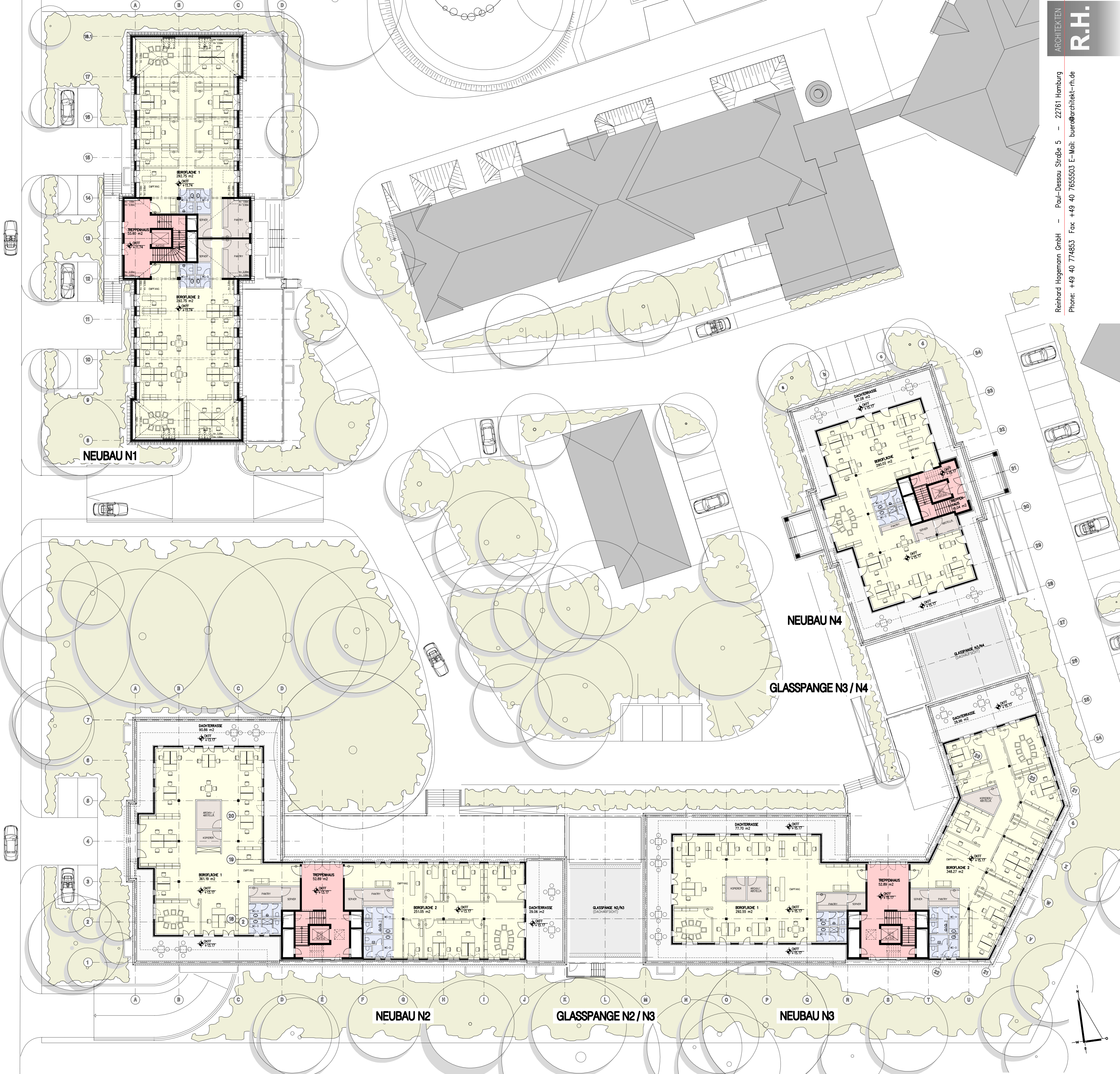
NEUBAU N1 - N4: GRUNDRISS DACHGESCHOSS ( N1 ) + STAFFELGESCHOSS ( N2 - N4 )
